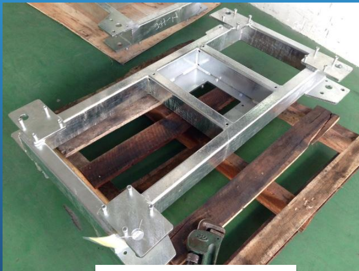
台車枠
